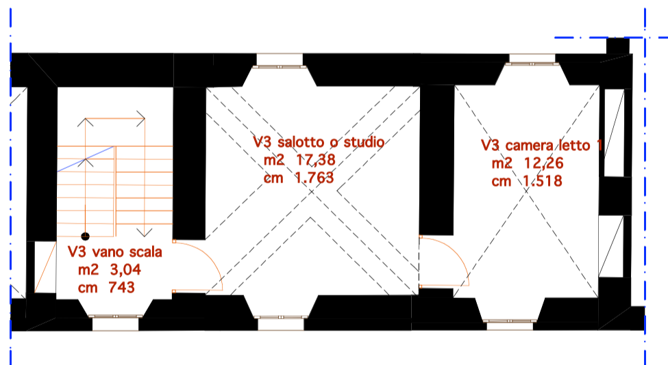
Piano primo
