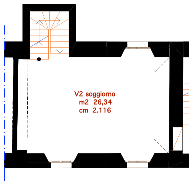
Piano primo
